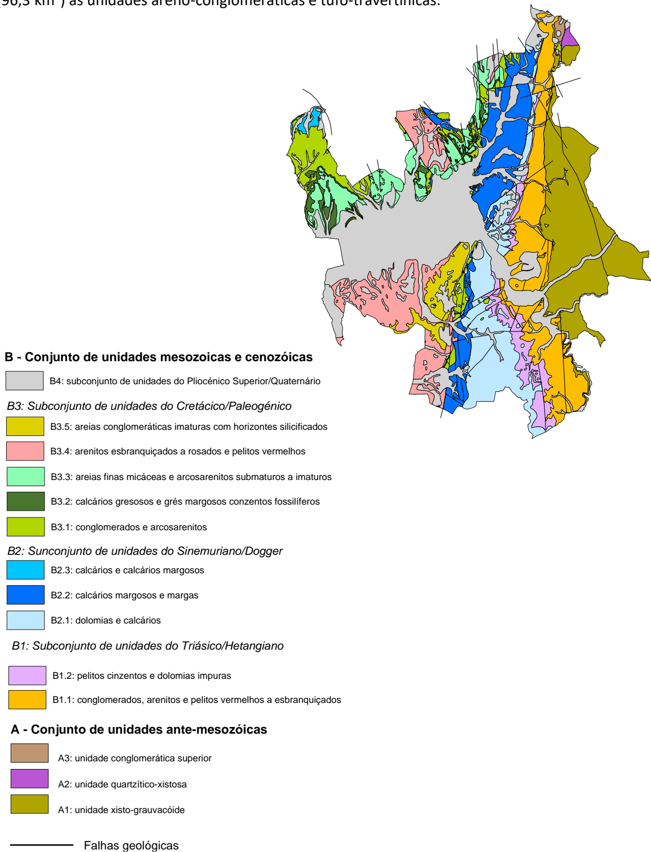
Figura 3.12 – Esboço Geológico
